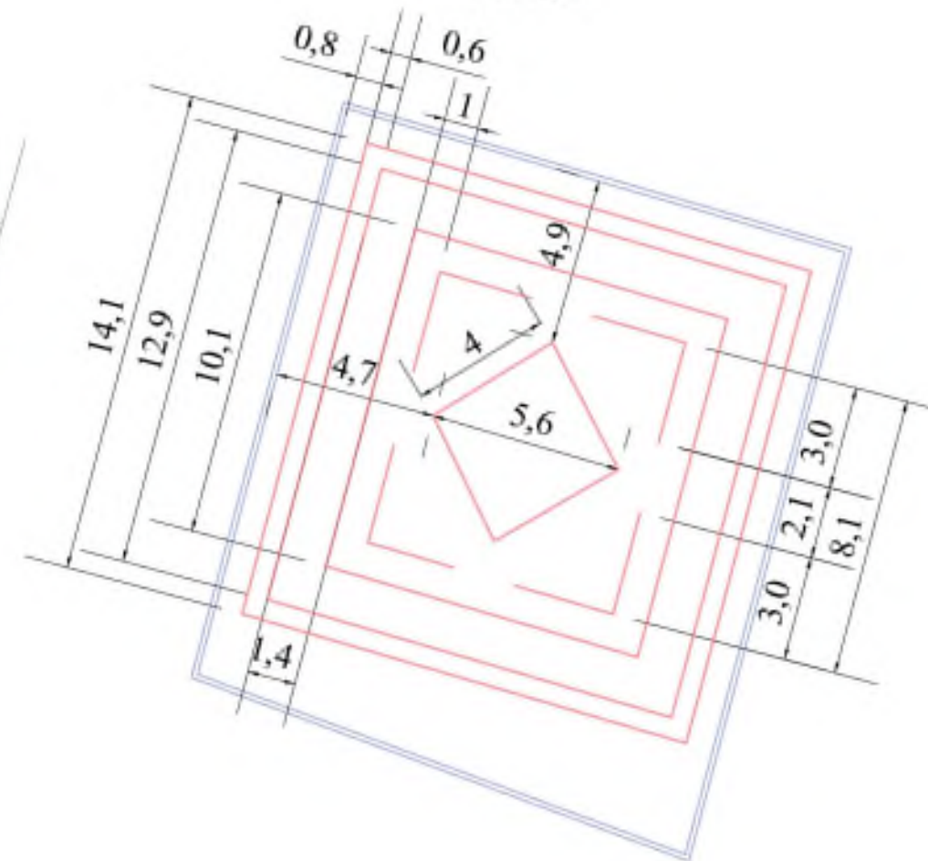
Разбивочный чертеж металлической отбортовки Цветников № 4.2, № 4.4 М 1:200
