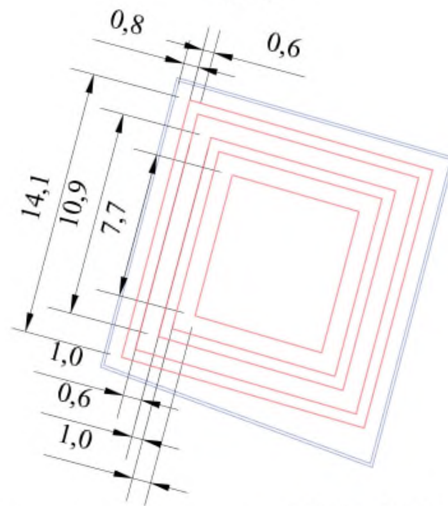
Разбивочный чертеж металлической отбортовки Цветников № 4.1, № 4.3, № 4.5 М 1:200
